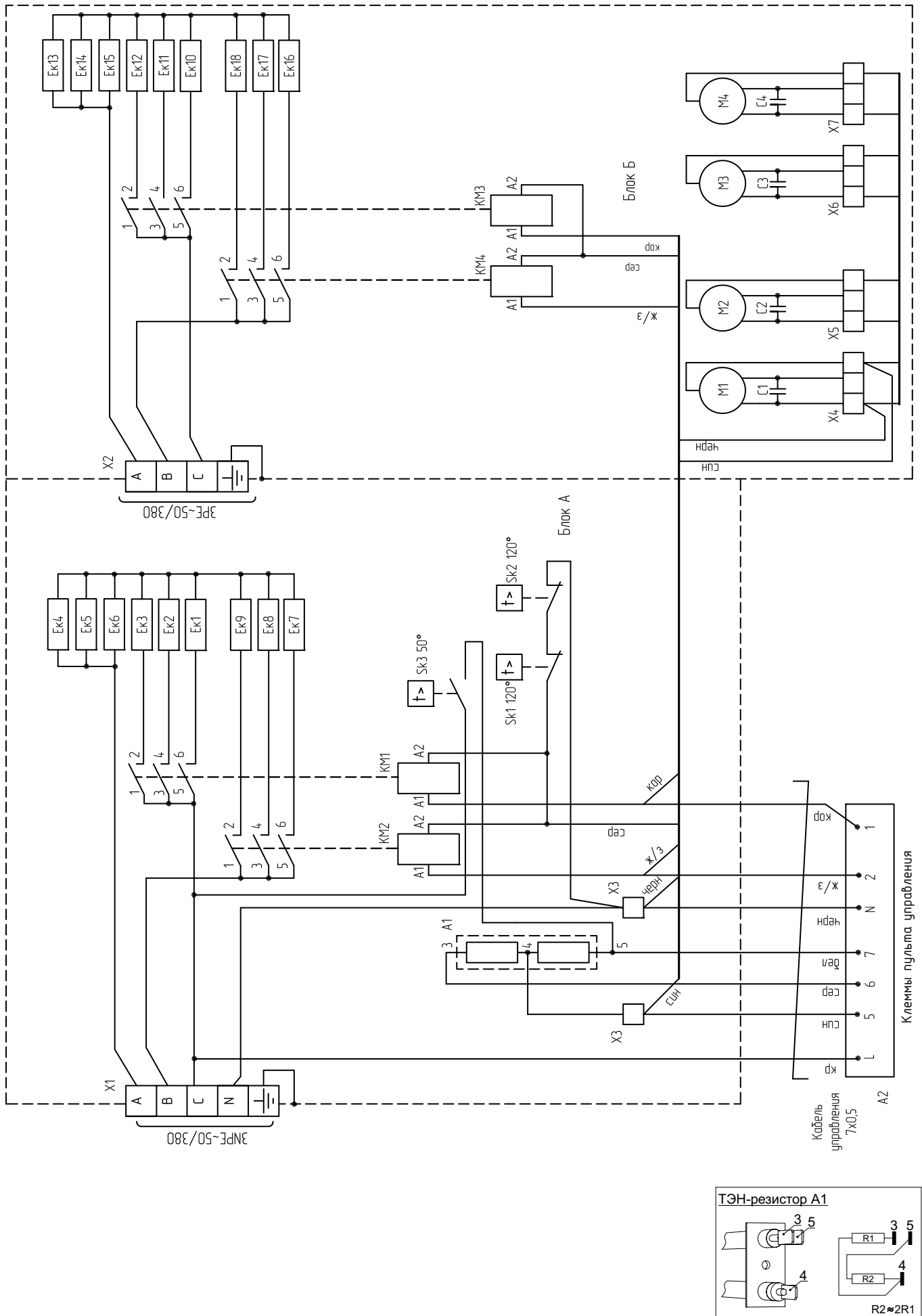
Рисунок 8. Электрическая схема занесы КЭВ-36;45П5032Е, КЭВ-54П5042Е
