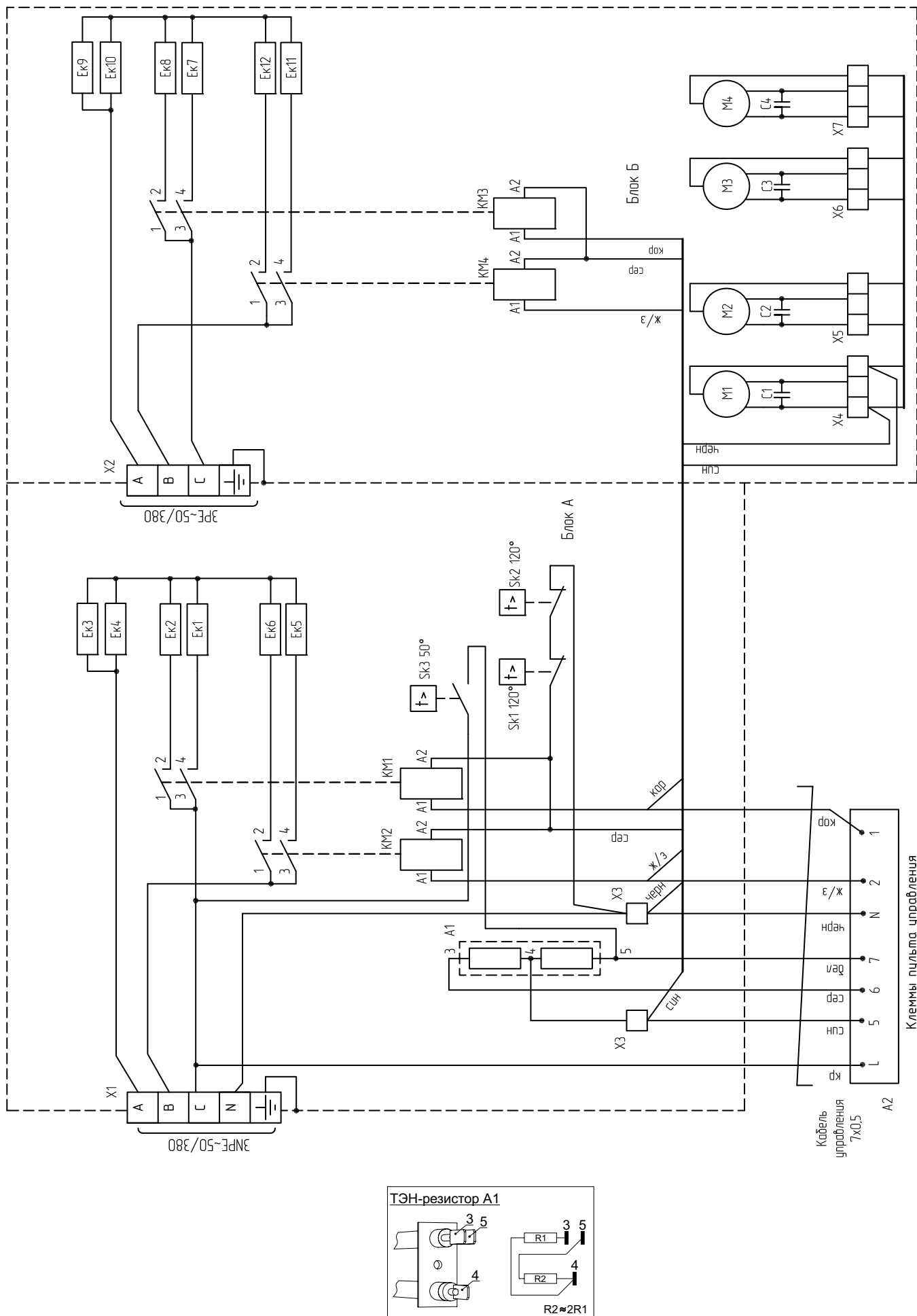
Рисунок 7. Электрическая схема занесы КЭВ-24;36П5042Е
