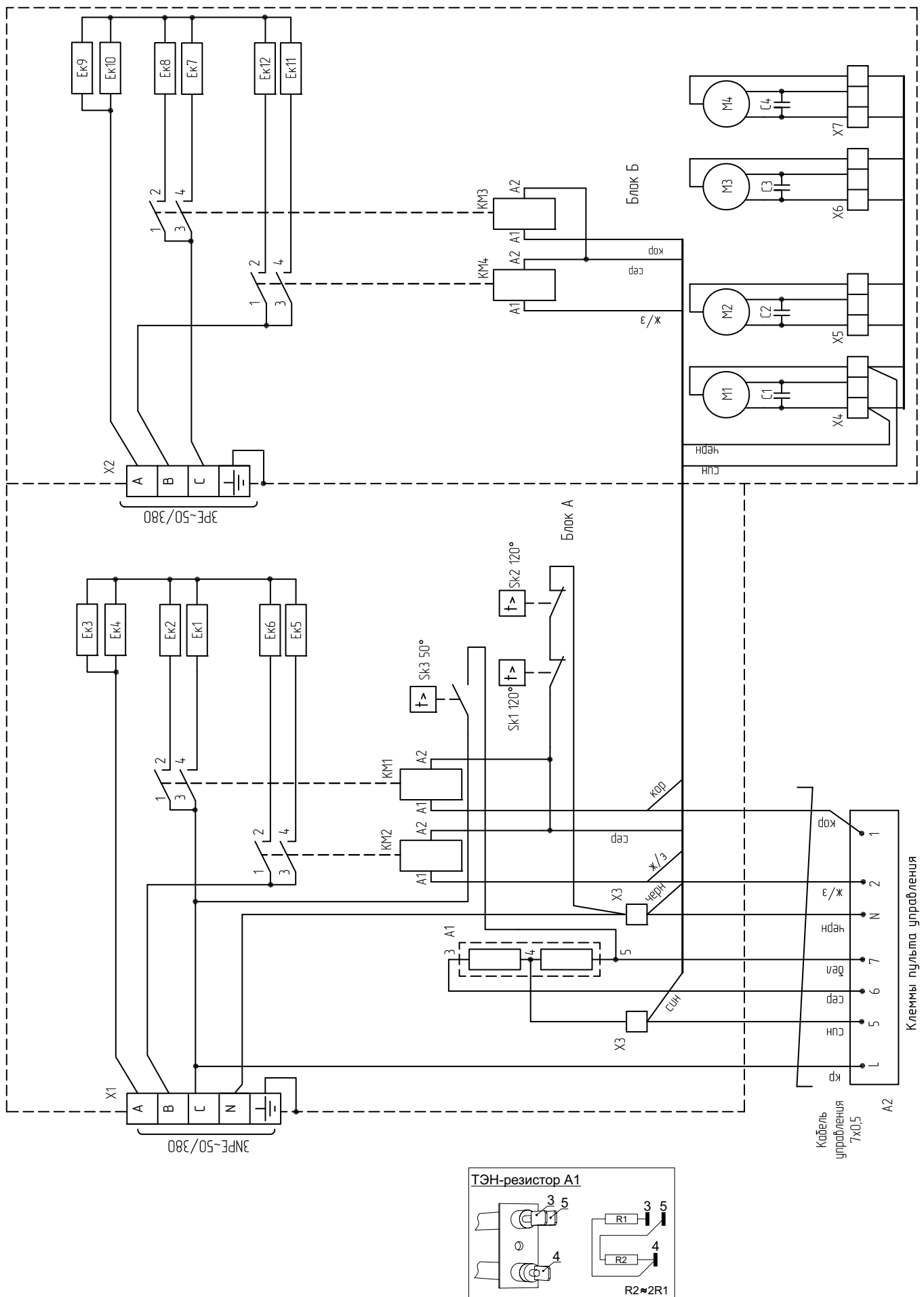
Рисунок 6. Электрическая схема завесы КЭВ-24П5032Е
